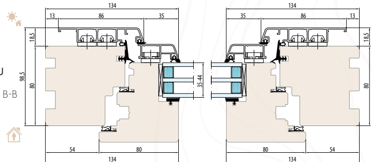
SYSTÈME NATURO 80 ALU GEMINI CLASSIC découpe pour l'appui de fenêtre extérieur
