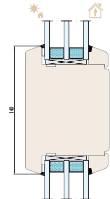
SYSTÈME NATURO 92 meneau structurel 140 mm
